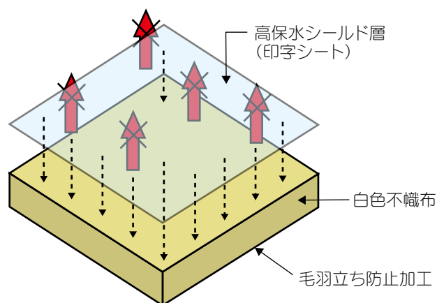
▲コンマツトWの層構造図
